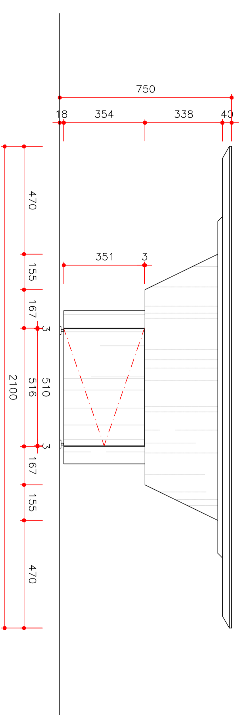
Zijaanzicht
