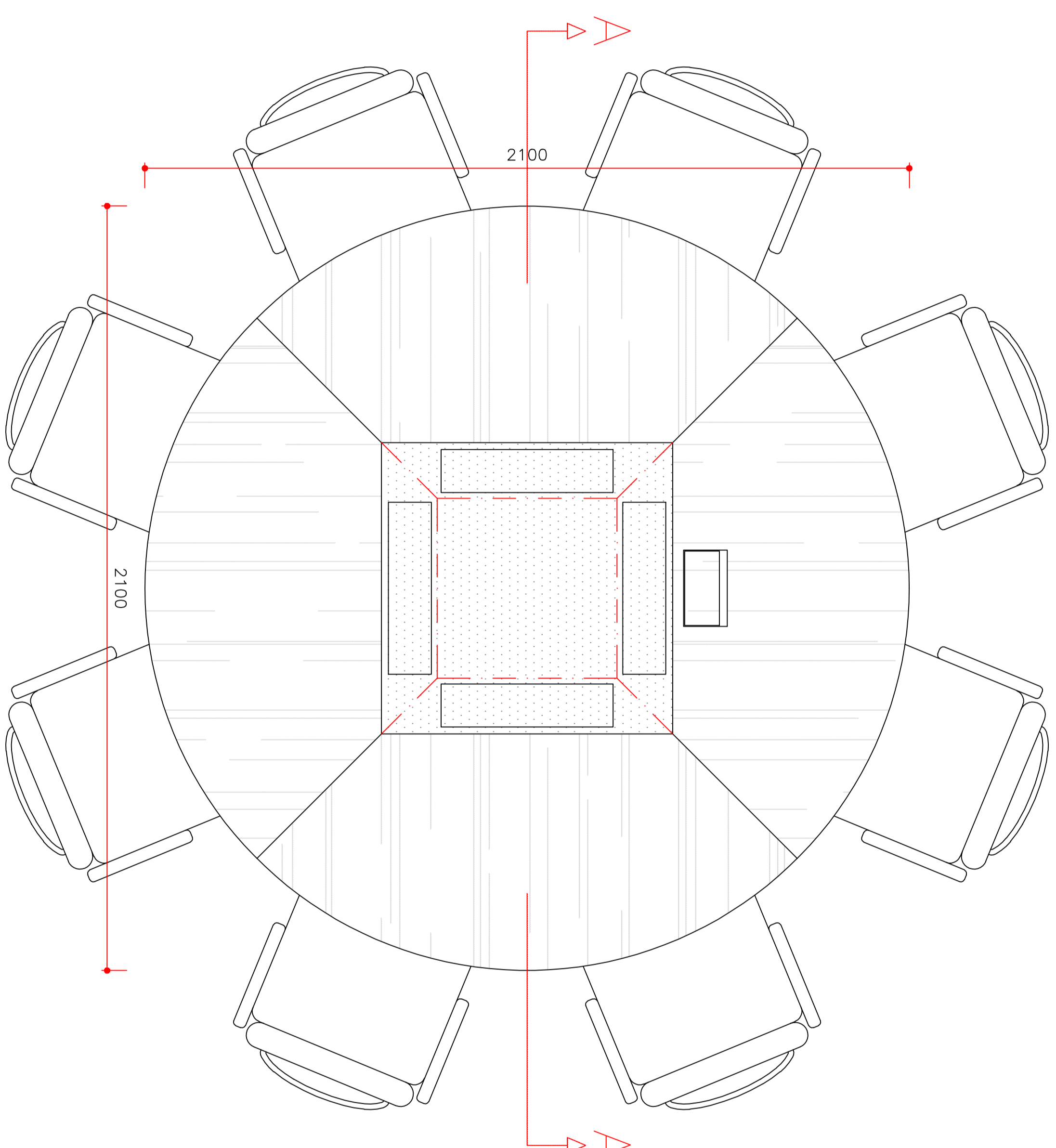
Bovenaanzicht
